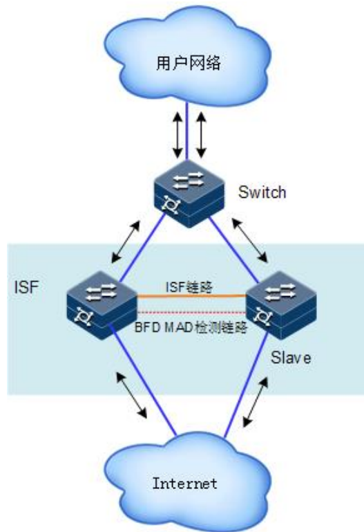
图3-10 BFD MAD 检测组网示意图（不使用中间设备）
