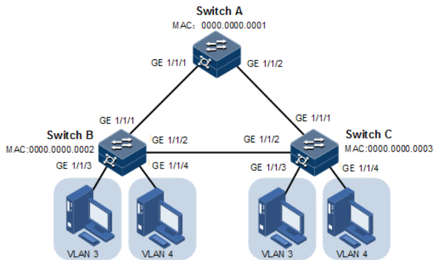
图2-18 MSTP 应用组网示意图
