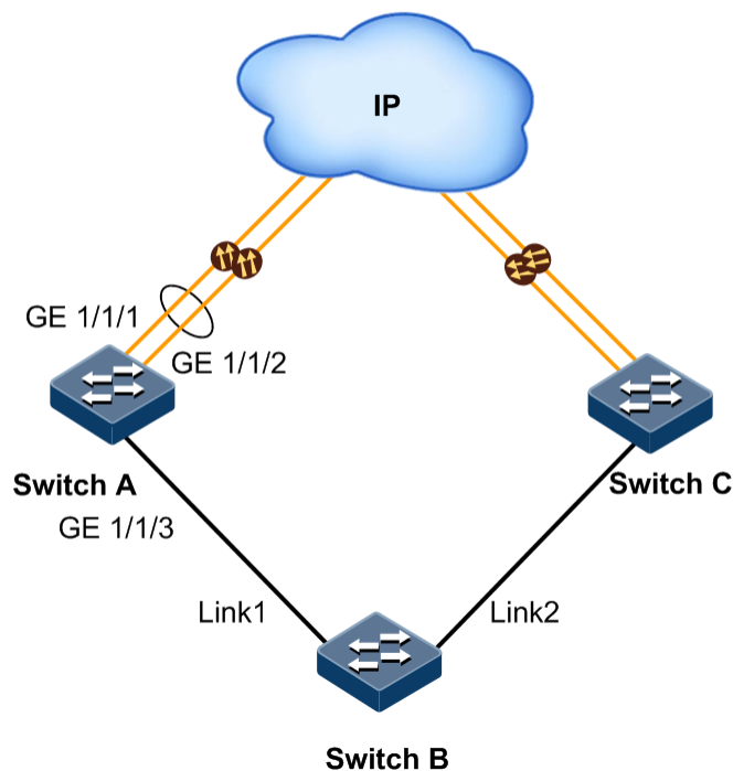
图12-5 故障转移应用组网示意图
