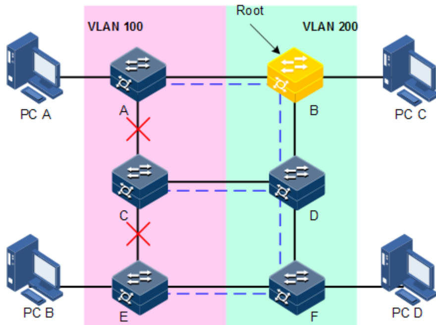
图2-13 RSTP 协议造成 VLAN 报文无法转发示意图
