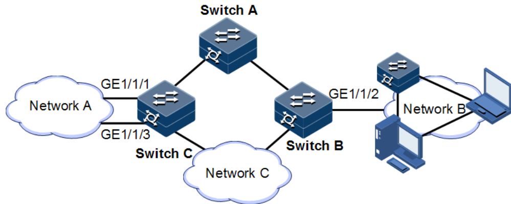
图2-19 环路类型示意图
