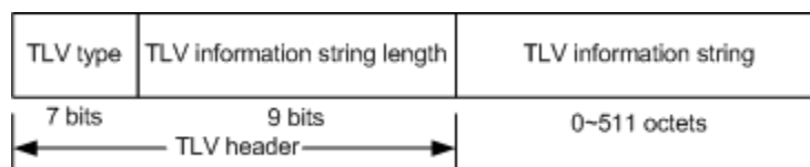
图13-8 基本 TLV 结构图
