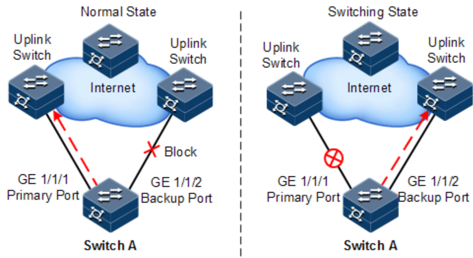
图12-2 接口备份原理示意图
