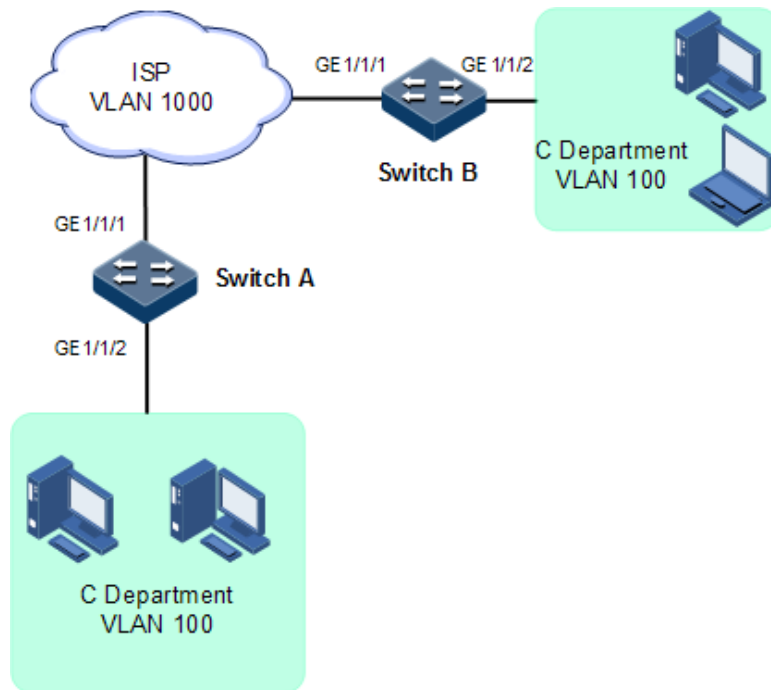
图2-7 基本 QinQ 应用组网示意图
