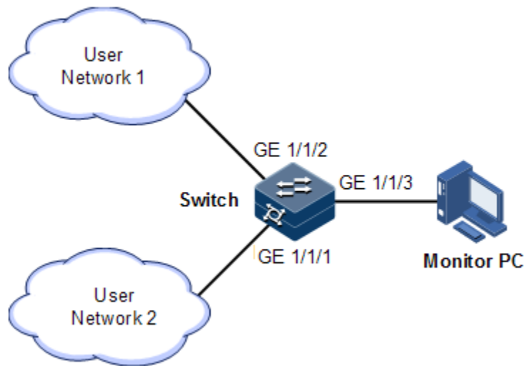
图2-23 接口镜像应用组网示意图
