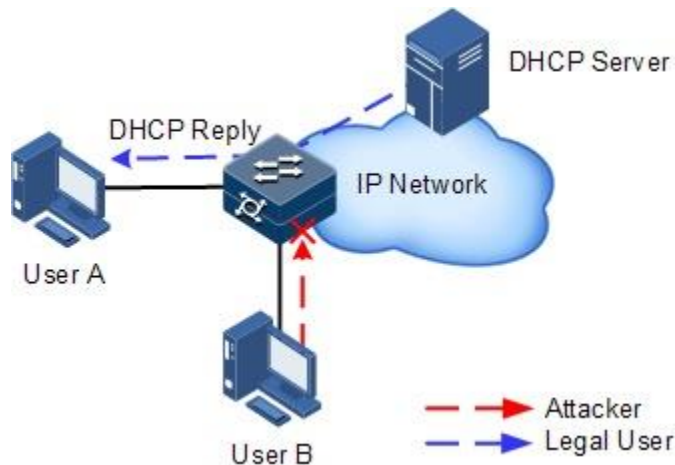
图11-9 IP Source Guard 功能示意图
