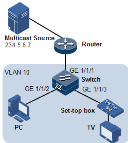
图9-7 IGMP Snooping 应用组网图
