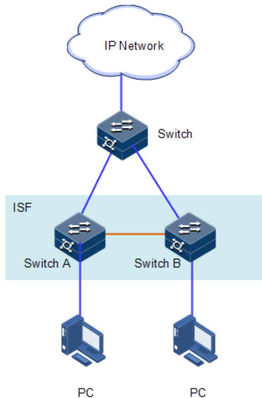
图3-1 ISF 组网应用示意图
