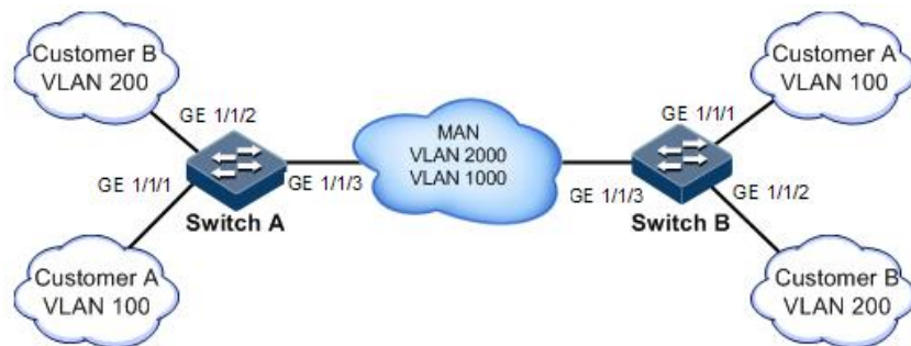
图2-24 配置 L2CP 功能组网示意图
