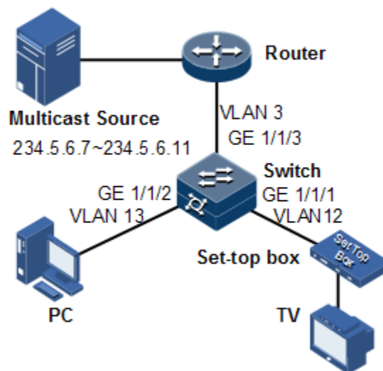
图9-10 接口下应用 IGMP 过滤组网图
