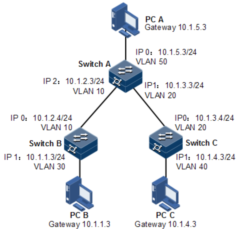
图5-5 配置静态路由组网示意图
