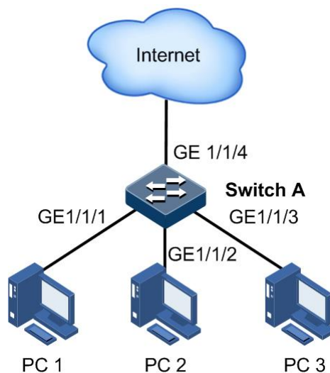
图2-21 接口保护组网示意图
