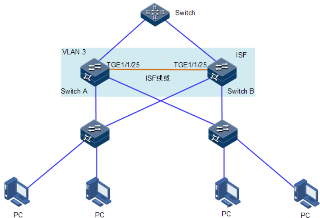
图3-16 ISF 典型配置组网图（BFD MAD 检测方式）
