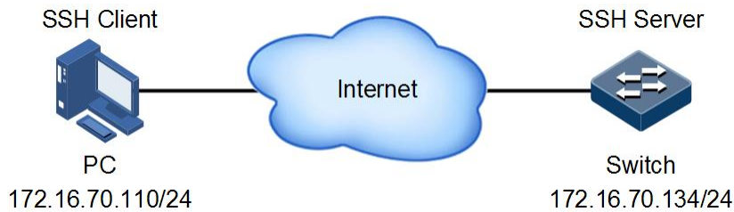
图1-6 SSH 登录设备组网示意图
