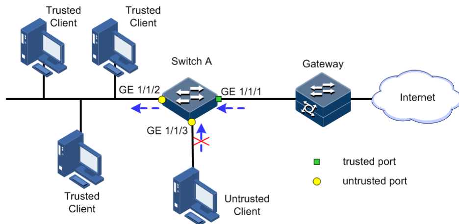
图5-8 配置 ND Snooping 组网示意图
