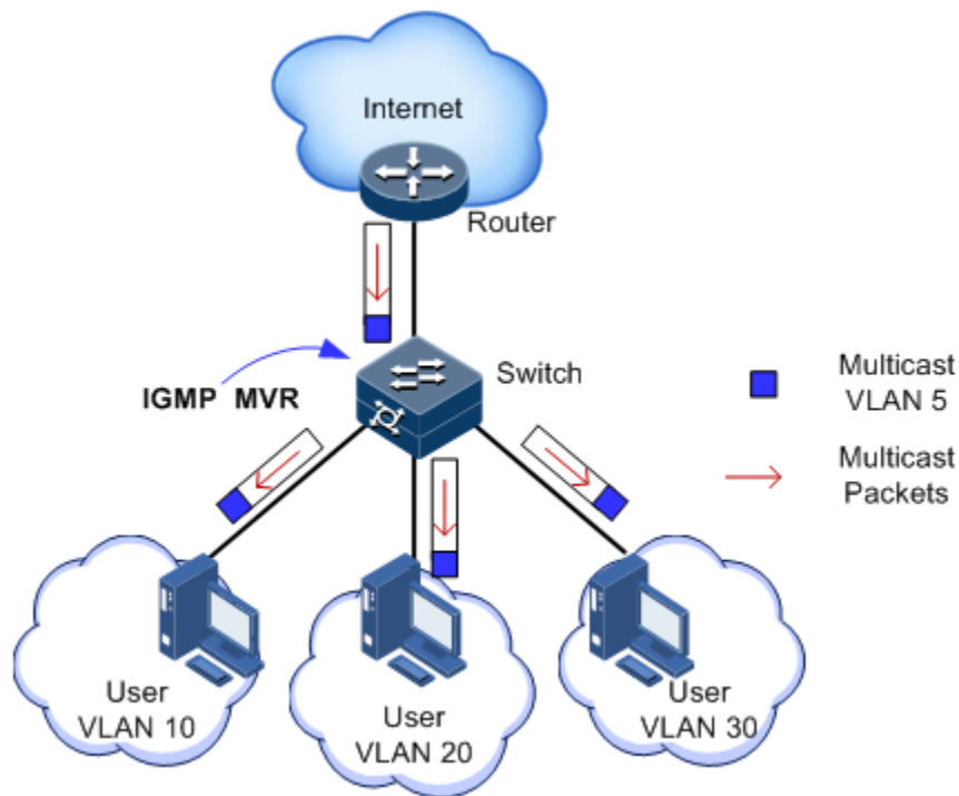
图9-11 IGMP MVR 数据传输示意图
