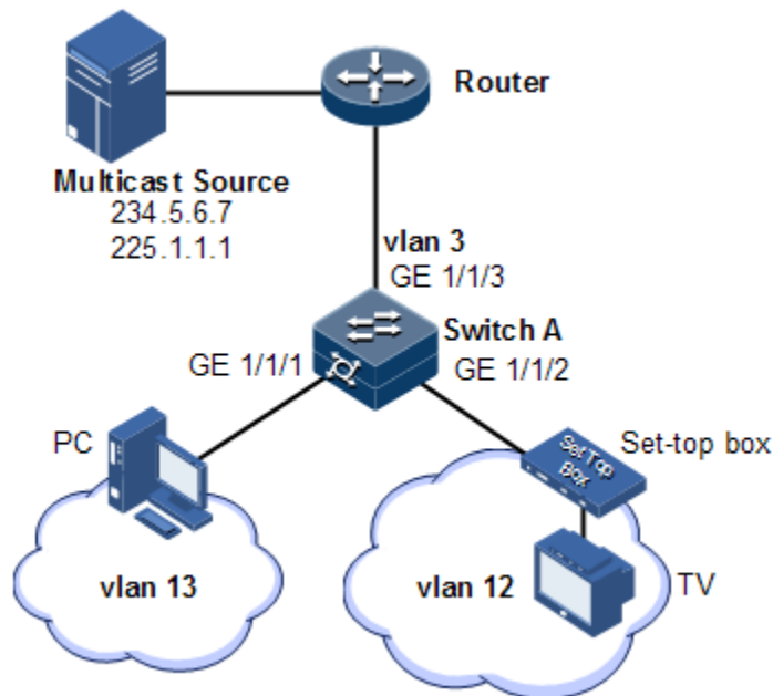
图9-9 IGMP MVR 应用组网图
