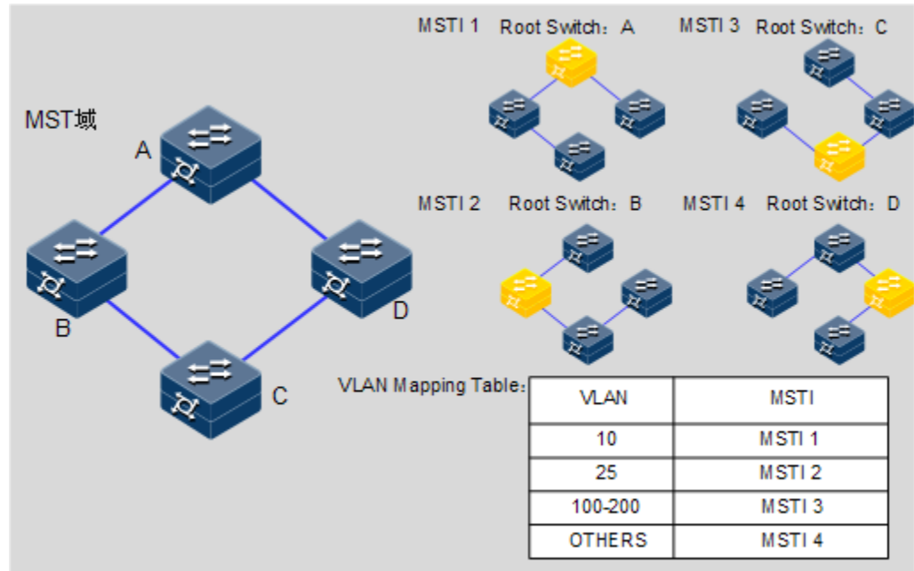
图2-16 MSTI 概念示意图
