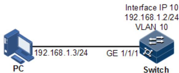
图5-1 配置 VLAN 接口组网示意图
