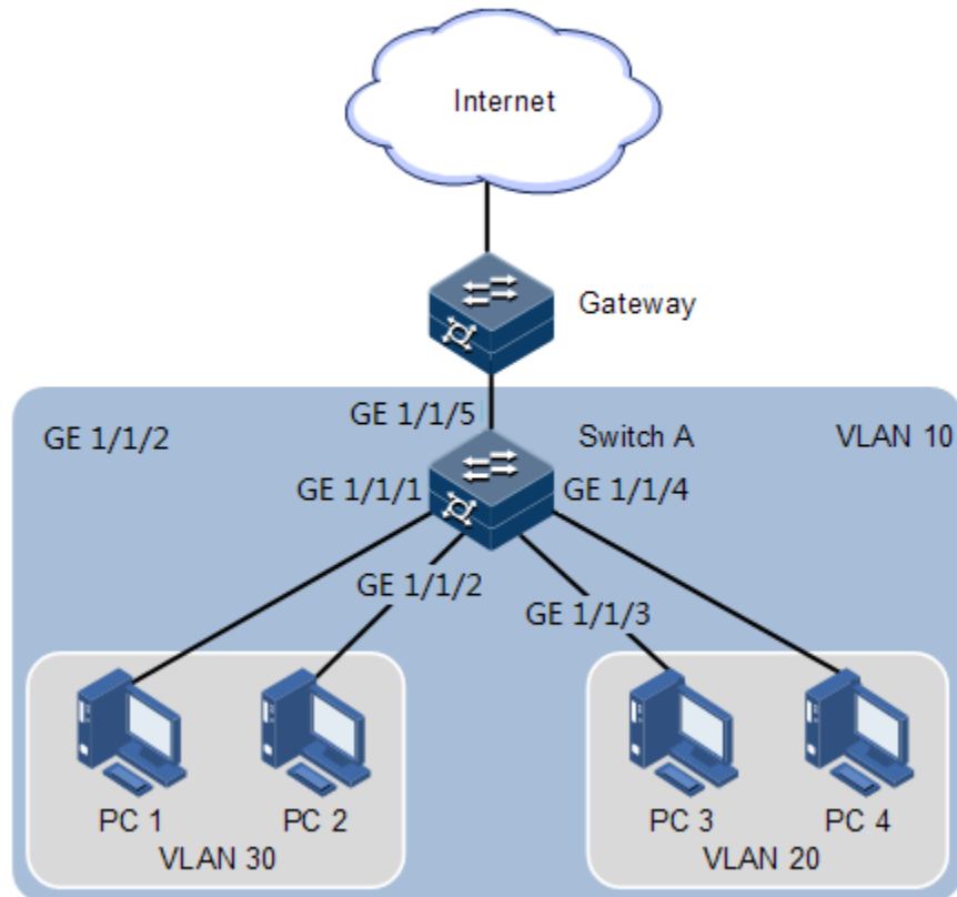
图2-5 PVLAN 应用组网示意图
