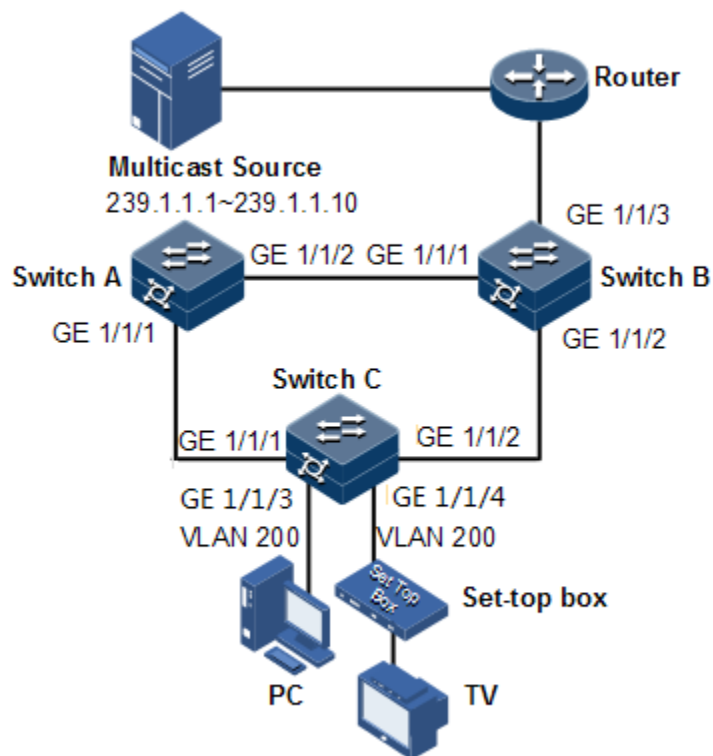
图9-6 环网上组播应用组网图
