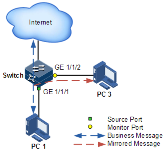
图2-22 接口镜像功能原理示意图
