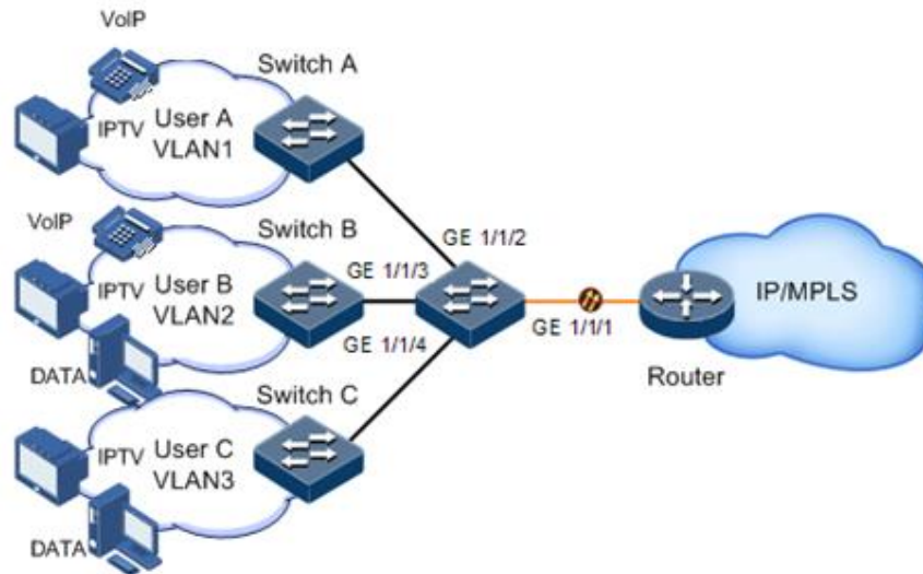
图8-10 配置基于流策略的流量限速组网示意图
