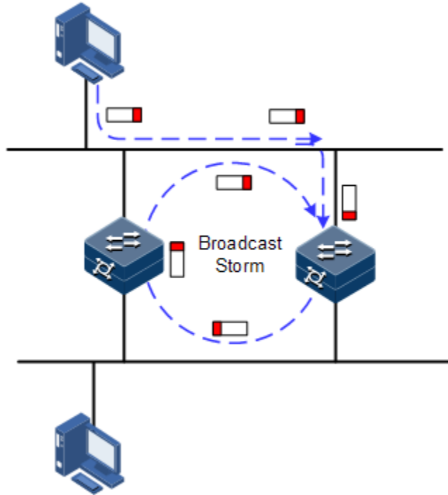
图2-11 网络环路造成网络风暴示意图
