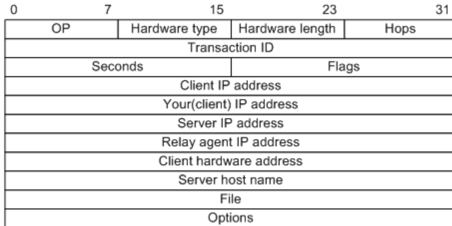
图7-12 DHCP 报文结构示意图
