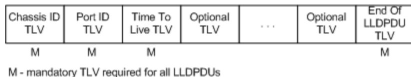
图13-7 LLDPDU 结构图
