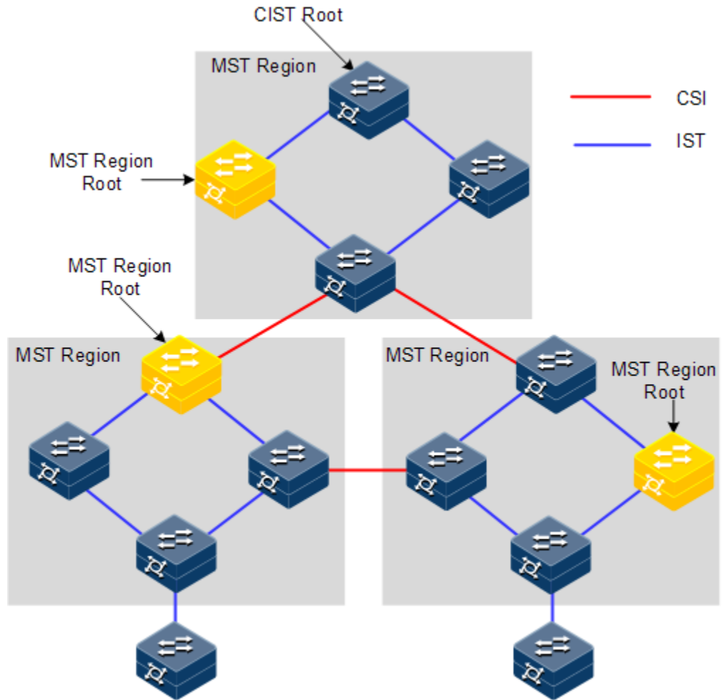
图2-15 MSTP 网络基本概念示意图
