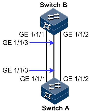
图12-1 静态 LACP 方式链路聚合应用组网示意图
