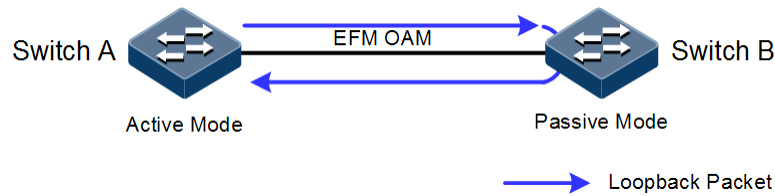
图10-1 OAM 环回示意图
