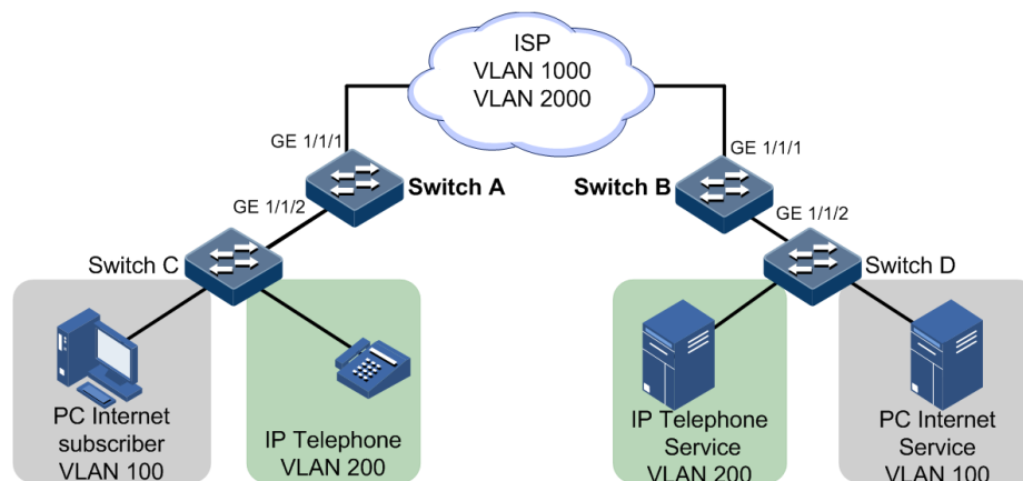
图2-8 灵活 QinQ 应用组网示意图
