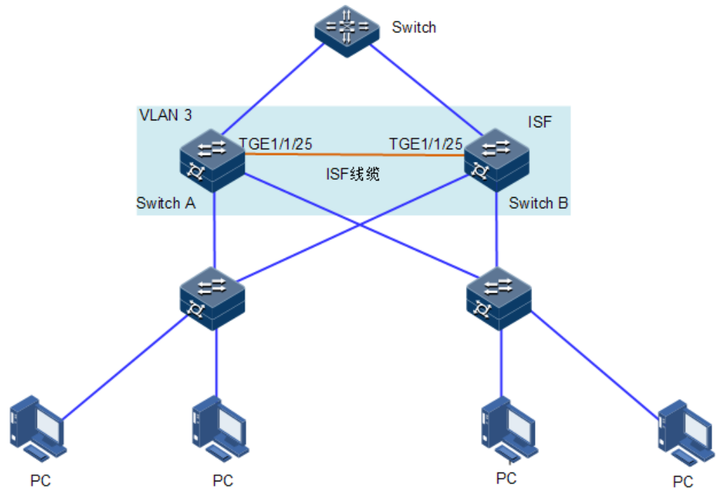
图3-15 成员设备从 ISF 模式恢复到独立运行模式组网图
