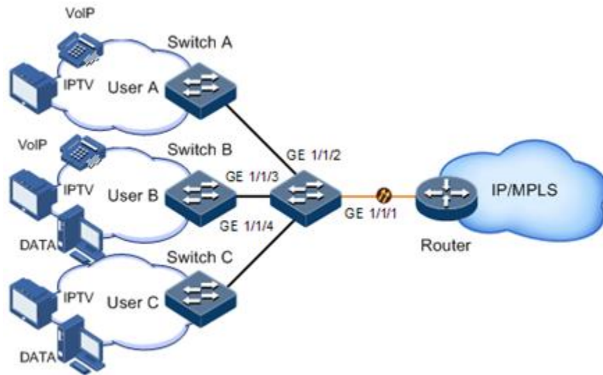
图8-11 配置基于接口的流量限速组网示意图
