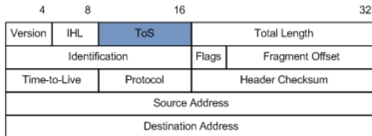
图8-2 IP 报文头部结构示意图
