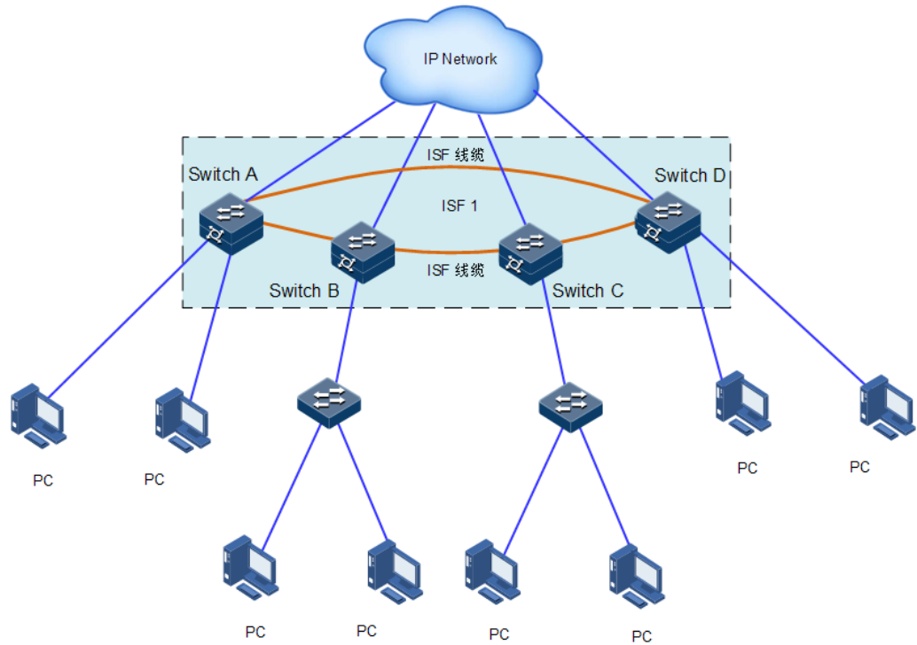
图3-18 将 Device A 改为 ISF 后的组网图
