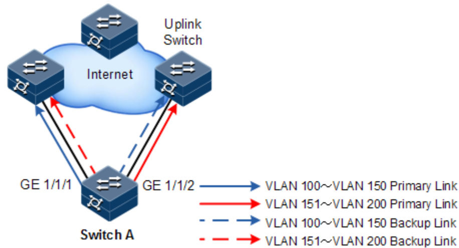
图12-3 接口备份在不同 VLAN 上的应用原理示意图
