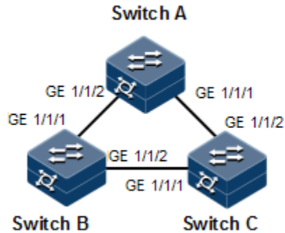
图2-14 STP 应用组网示意图
