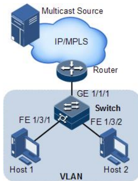
图9-5 IGMP Snooping 应用场景
