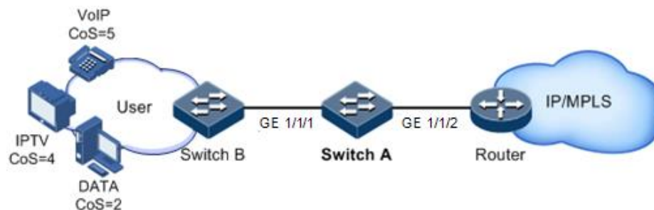
图8-9 配置队列调度组网示意图
