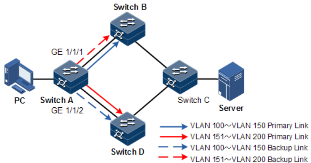
图12-4 接口备份应用组网示意图
