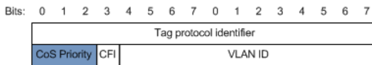
图8-5 CoS 优先级报文结构示意图
