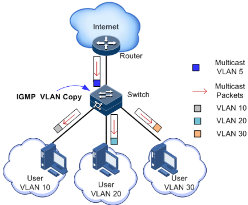
图9-12 组播 VLAN 复制数据传输示意图
