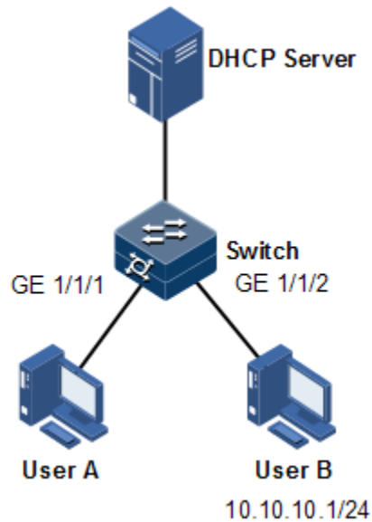
图11-10 IP Source Guard 应用组网示意图
