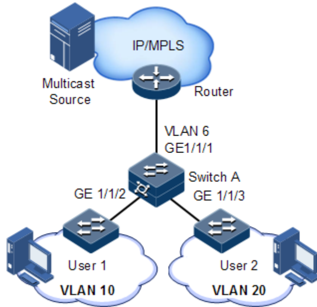
图9-13 组播 VLAN 复制应用场景
