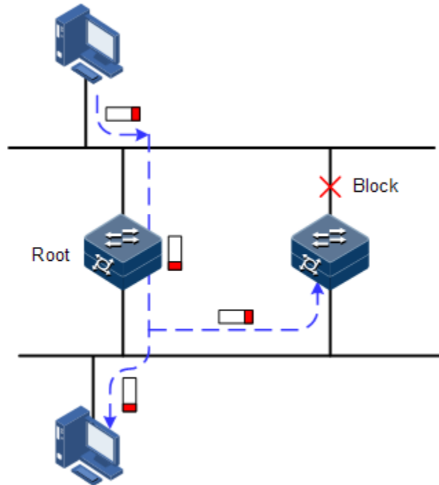
图2-12 运行 STP 协议的环网示意图
