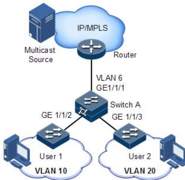
图9-8 IGMP MVR 应用场景
