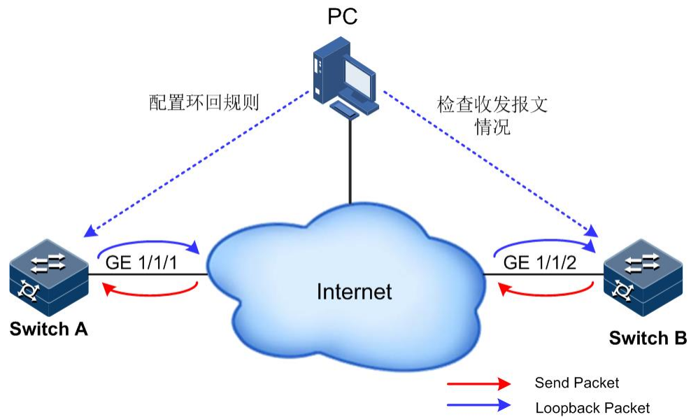
图5-2 接口环回示意图
