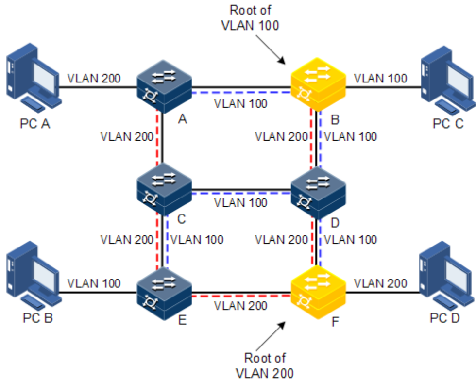
图2-17 MST 域内多生成树实例组网示意图
